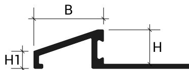
ZRM 80 - Aluminum
